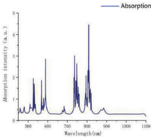
Nd: YAG吸收光谱
